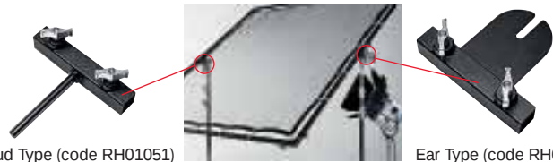
Stud Type (code RH01051)
